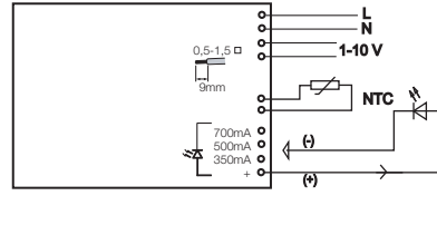
Circuit diagram A: 1-10V ⊙
